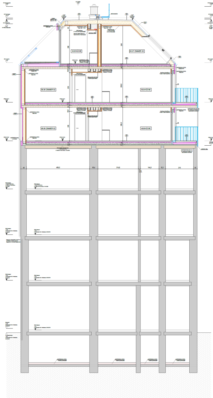
SCHNITT A-A
