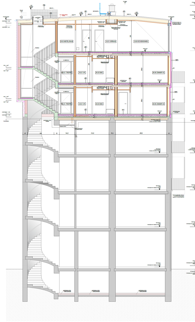
SCHNITT B-B
